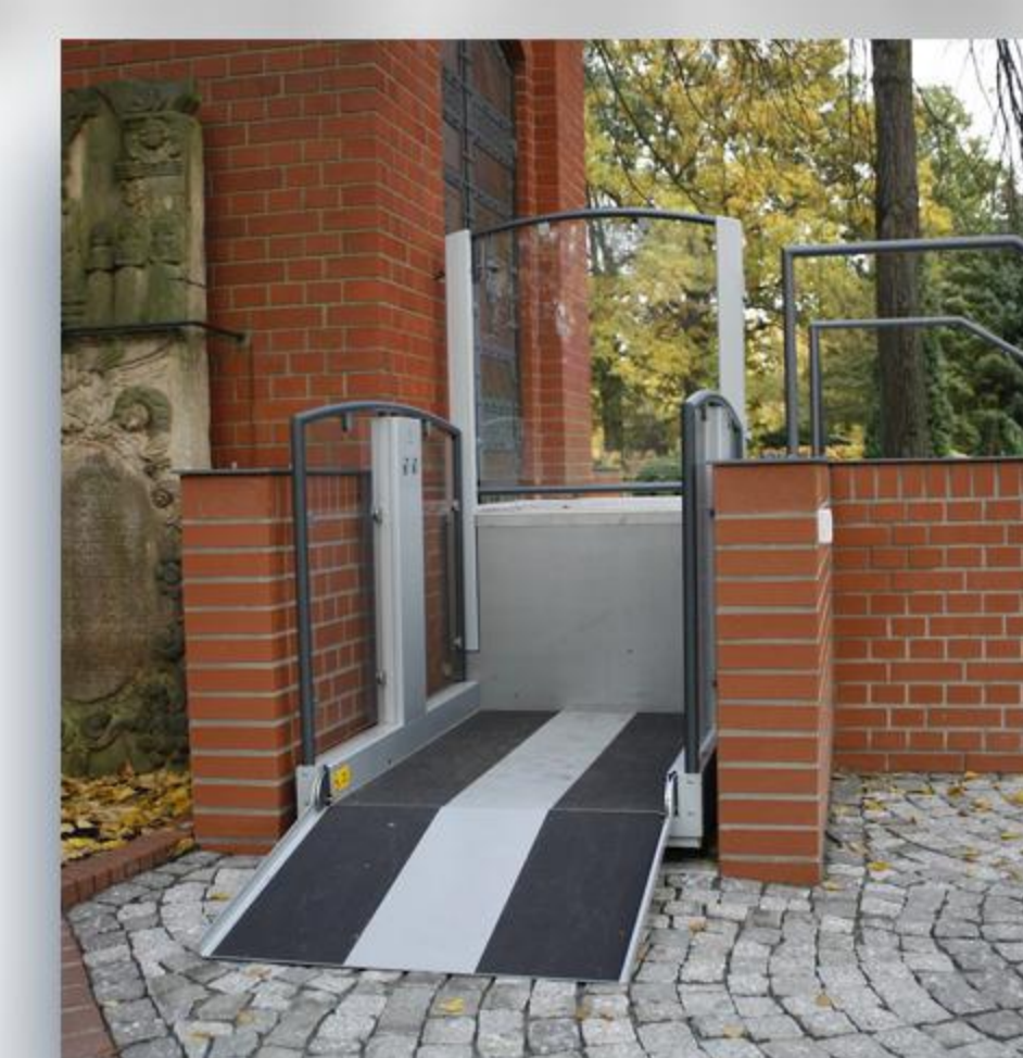
LP5+ Hebeplattform Hubhöhe bis 830mm
