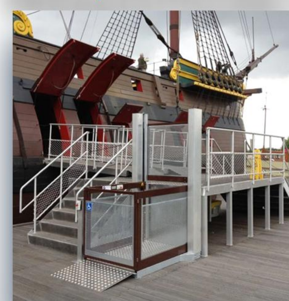
LP8 Hebeplattform Hubhöhe bis 3m
